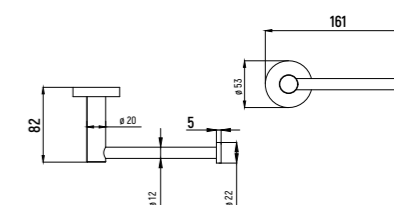
ДЕРЖАТЕЛЬ ТУАЛЕТНОЙ БУМАГИ — AQM7208
