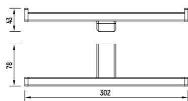
ДЕРЖАТЕЛЬ ТУАЛЕТНОЙ БУМАГИ ДВОЙНОЙ
