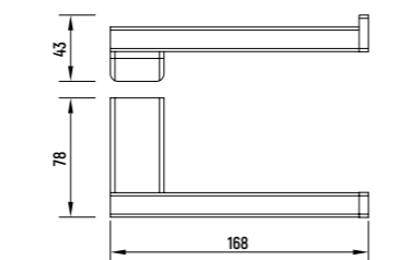
ДЕРЖАТЕЛЬ ТУАЛЕТНОЙ БУМАГИ
