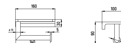
ДЕРЖАТЕЛЬ ТУАЛЕТНОЙ БУМАГИ С ПОЛКОЙ — AQM7209
