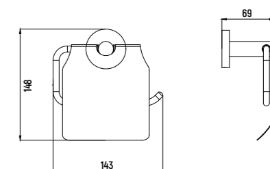
ДЕРЖАТЕЛЬ ТУАЛЕТНОЙ БУМАГИ С КРЫШКОЙ — AQM7210
