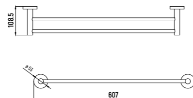
ДЕРЖАТЕЛЬ БАННОГО ПОЛОТЕНЦА ДВОЙНОЙ — AQM7205
